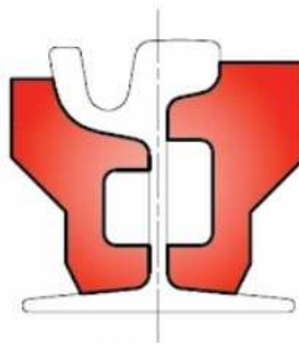
WERSJA 2 - "średnie" szyny: 60R1, 60R2, 59R1, 59R2
