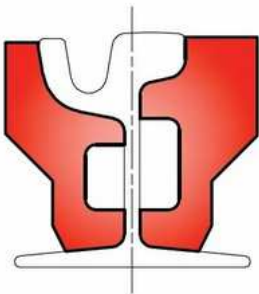
WERSJA 1 - "wysokie" szyny: 60R1, 60R2, 59R1, 59R2
